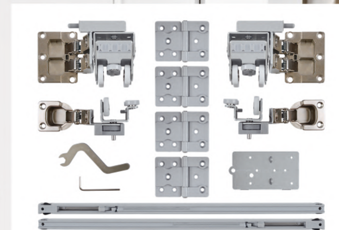
Комплект фурнитуры для одной складной двери
