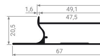
MZ 20 Профиль фасадный
