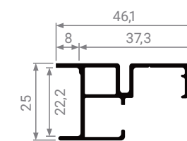
MT 902 N Нижняя направляющая
