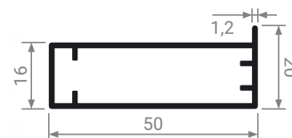
MZ 10 Профиль фасадный
