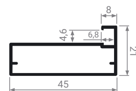
MZ 13 Профиль фасадный
