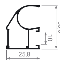
MS 120 Профиль вертикальный асимметричный
