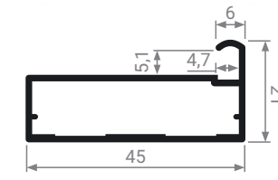
MZ 09 Профиль фасадный
