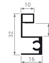
MS 213 Профиль горизонтальный верхний
