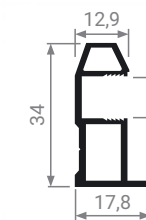
MS 161 Профиль вертикальный
