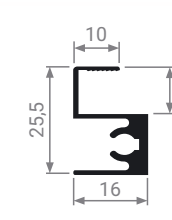
MS 215 Профиль горизонтальный верхний
