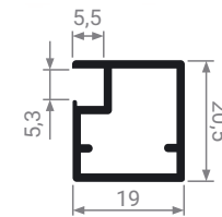
MZ 01 Профиль фасадный
