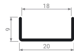
C18-02 Профиль фасадный
