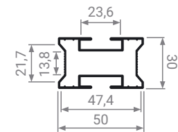
РА 01 Профиль опорный алюминиевый
