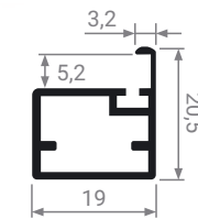
MZ 07 Профиль фасадный
