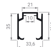
MS 184 Направляющая для подвесной системы
