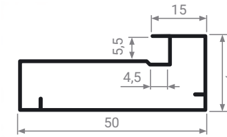
MZ 04 Профиль фасадный
