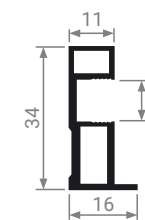
MS 163 Профиль вертикальный
