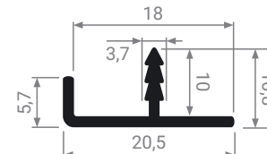
T 18-03 Профиль врезной
