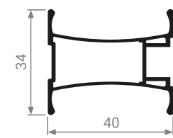
MS 155 Профиль вертикальный
