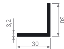
Уголок для крепления направляющей к стене
