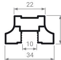
MS 160 Профиль вертикальный
