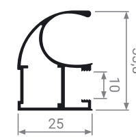
MS 125 Профиль вертикальный асимметричный
