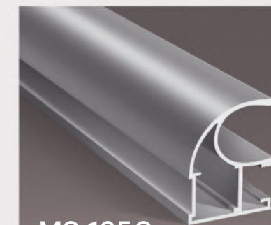
MS 125C Профиль вертикальный асимметричный Облегченная версии MS 125
