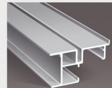
MT 902 N Нижняя направляющая
