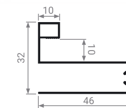
MS 223 Профиль горизонтальный нижний
