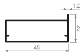
MZ 12 Профиль фасадный
