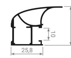
MS 130 Профиль вертикальный асимметричный
