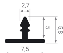
T-08 Профиль разделительный декоративный врезной
