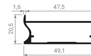
MZ 19 Профиль фасадный
