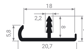
T 18-02 Профиль врезной
