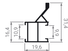
MS 145 Профиль вертикальный
