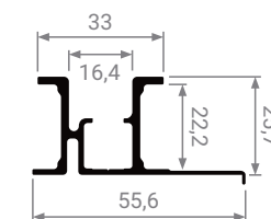
MT 902 V Верхняя направляющая
