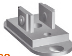
PP 02 Крепление пол-потолок с площадкой под саморез
