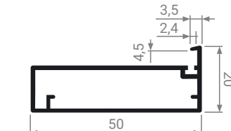
MZ 17 Профиль фасадный
