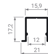
MS 185 Профиль врезной нижний для деревянных дверей
