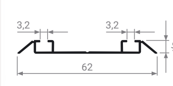
MS 320C Направляющая нижняя
