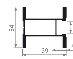
MS 170 Профиль вертикальный
