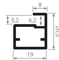
MZ 02 Профиль фасадный
