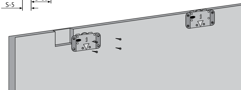
Схема установки роликов
