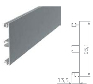
Цоколь алюминиевый 100
