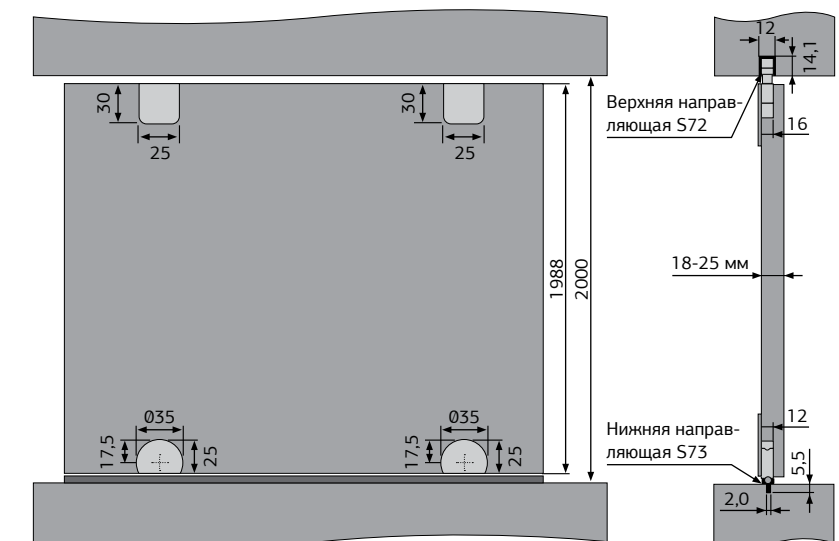
Схема фрезеровки фасада
