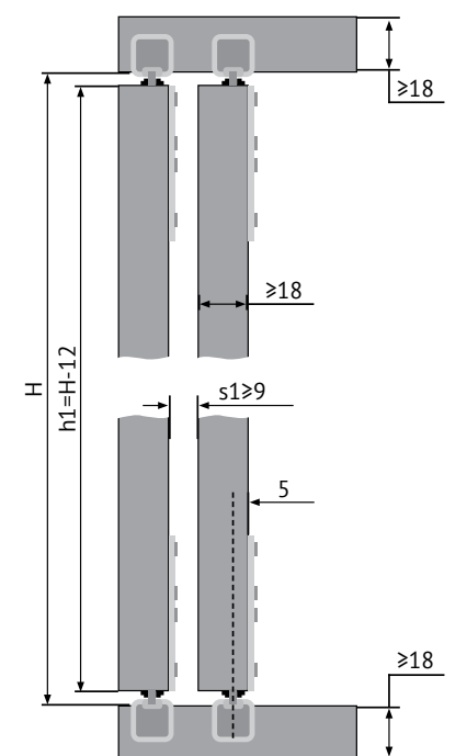
Схема расположения фасадов
