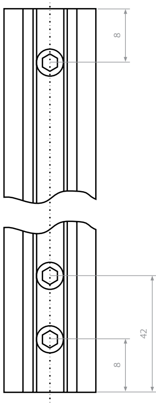
Присадка отверстий для раздвижных систем MS
