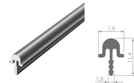
Направляющая нижняя S73
