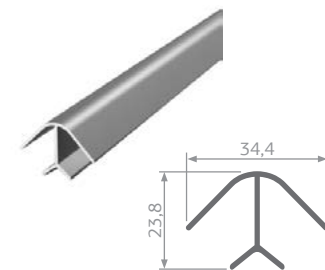
Угол универсальный
