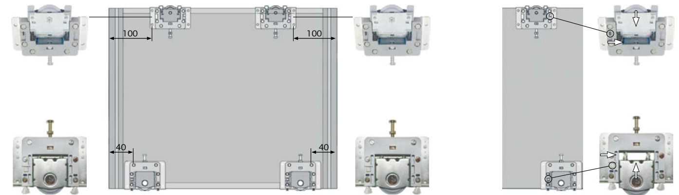
Схема установки роликов
