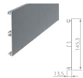
Цоколь алюминиевый 150
